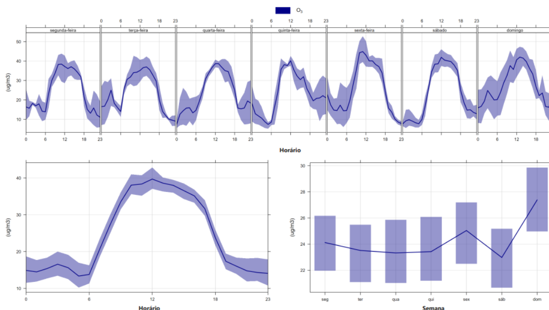
Figura 6.4.4-1: Evolução horária e semanal de O 3 da EAMQAR.
