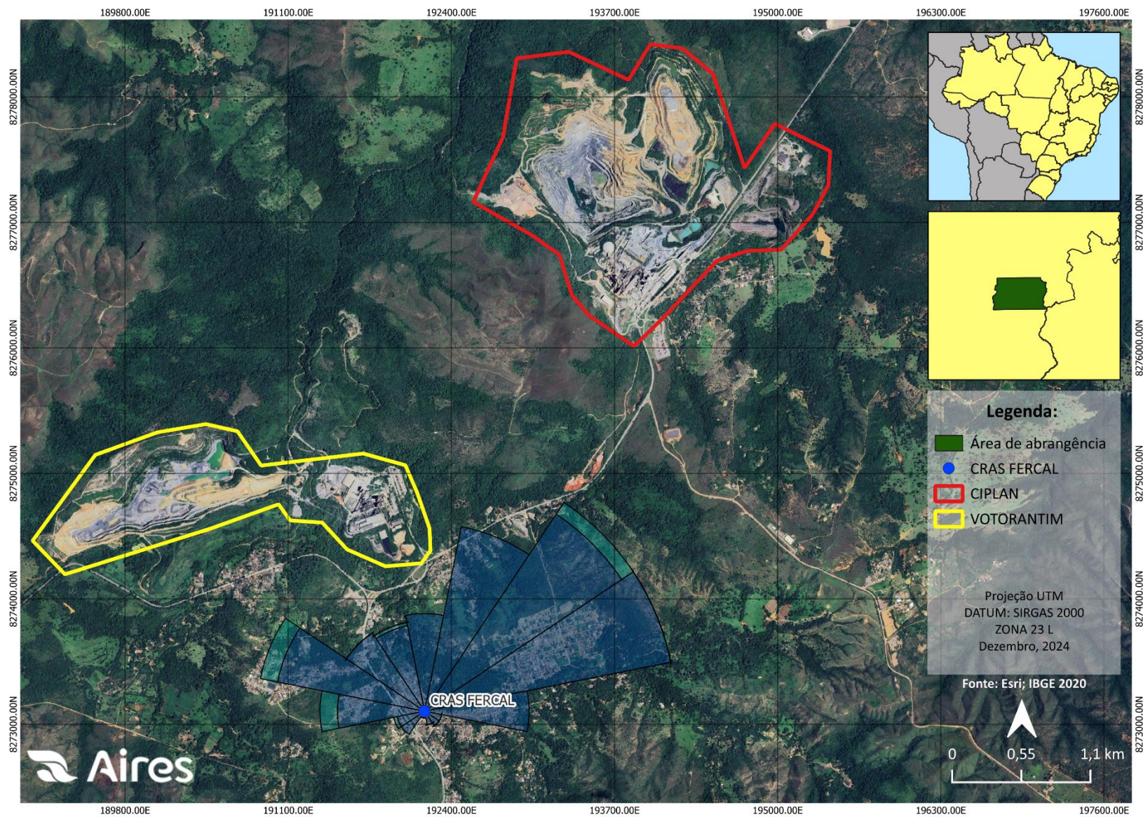
Figura 5.1-2: Localização do ponto e a rosa dos ventos referente ao mês de novembro de 2024.
