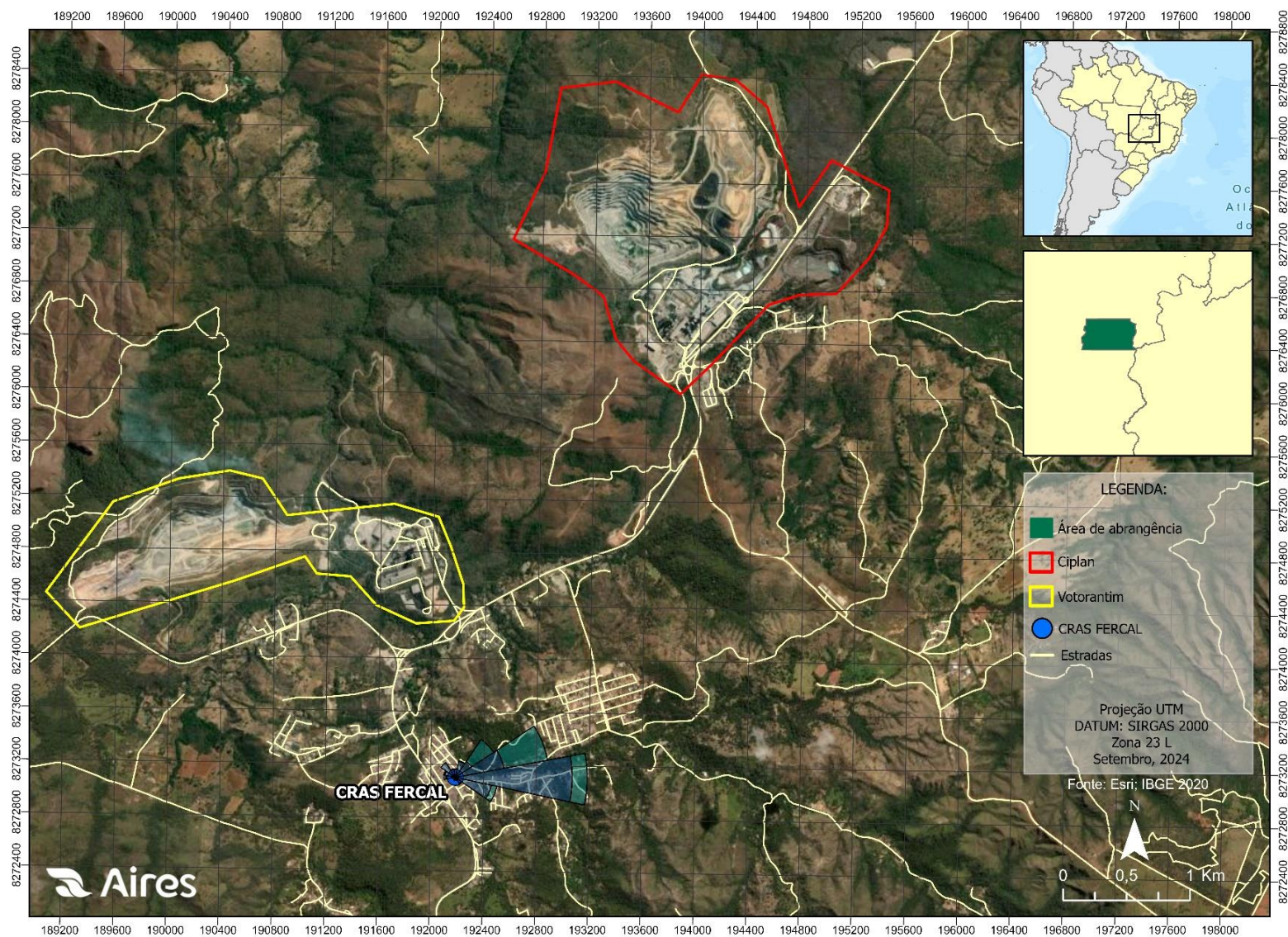
Figura 5.1-2: Localização do ponto e a rosa dos ventos referente ao mês de agosto de 2024.
