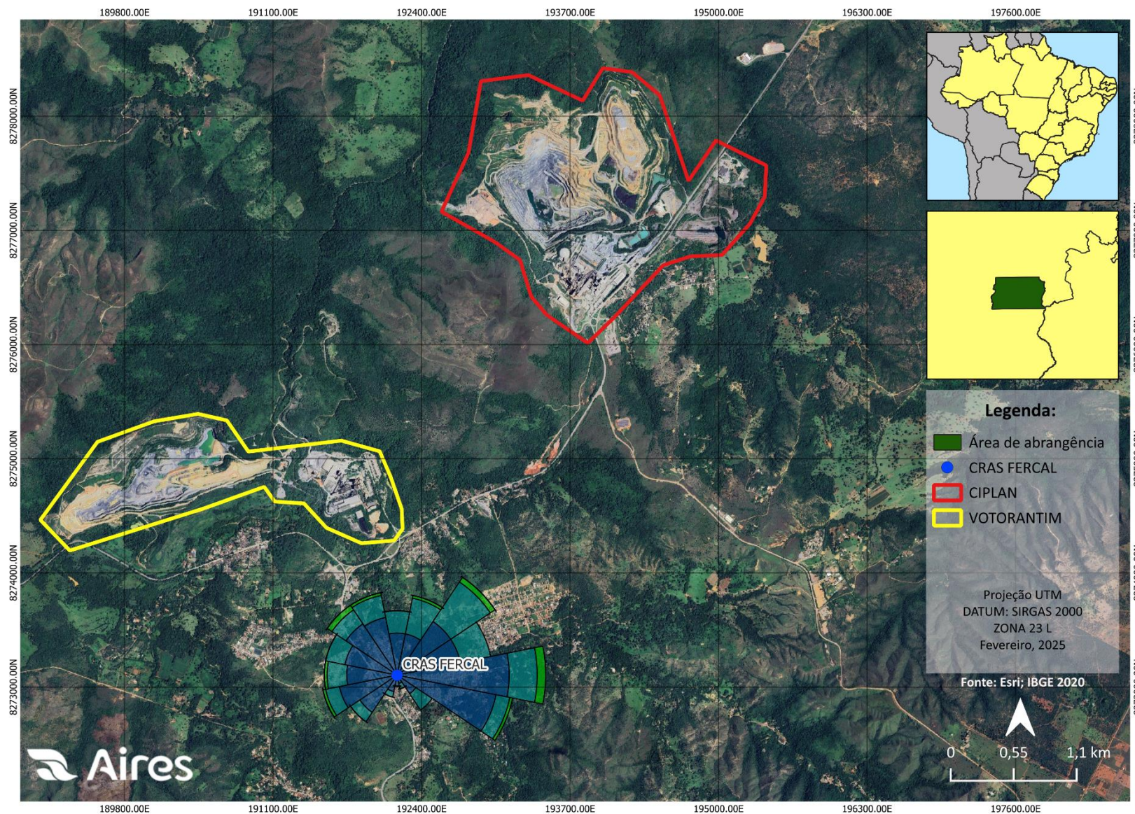
Figura 5.1-2: Localização do ponto e a rosa dos ventos referente ao mês de dezembro de 2024.
