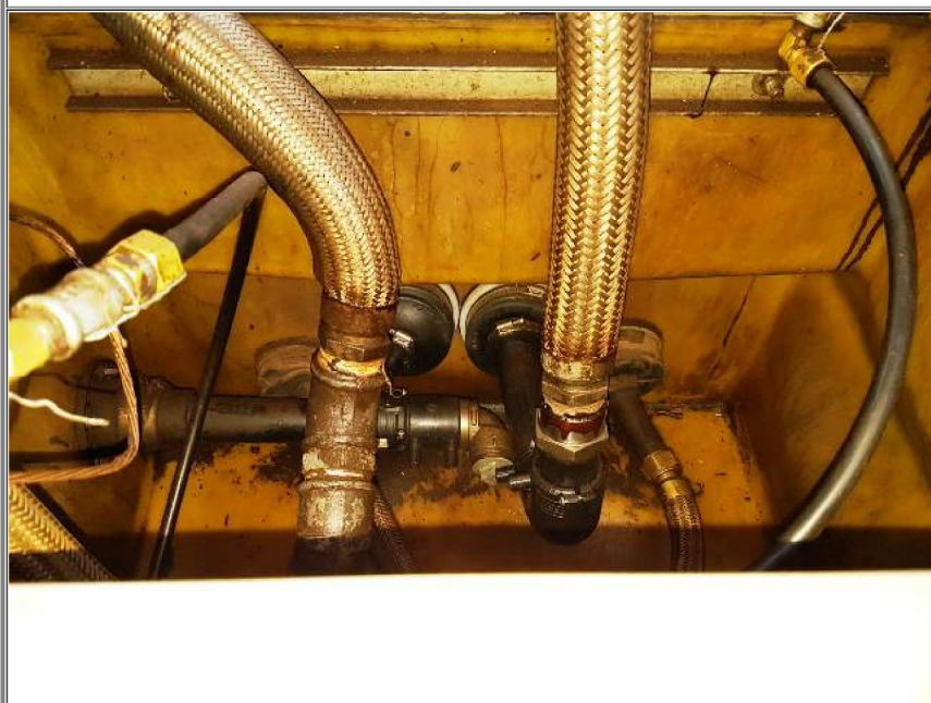
Foto 7 - Camara de contenção da bomba cercando todo o equipamento com checkvalve
