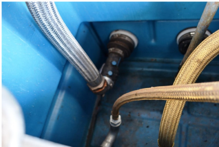
Figura 5 - Detalhe interno da Câmara de contenção de uma das Unidades Abastecedoras do SASC. Observa-se que a tubulação está totalmente contida no sump da câmara de contenção no dispositivo de segurança. Os sumps das demais unidades necessita de manutenção operacional diária conforme exige a tabela 1 da ABNT NBR 15594-3:2008
